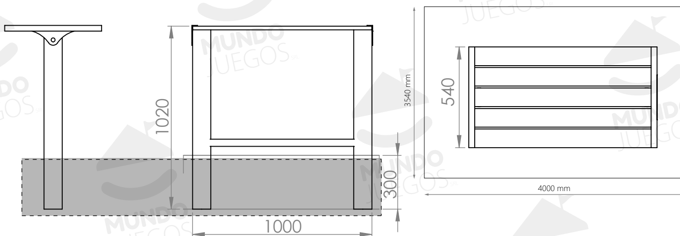
Vista lateral
